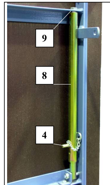
Fig. 46 Schuifbuis vario-platform
