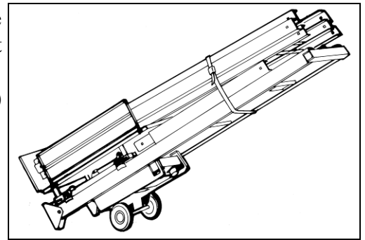
Fig. 12 Verrijdbaar onderstel
