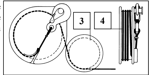
Fig. 65 PVC-plaatje kabelmontage
