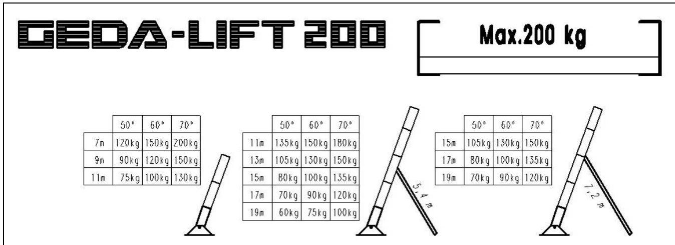
Fig. 24 Belastingtabel voor ladderdelen 150/200 kg
