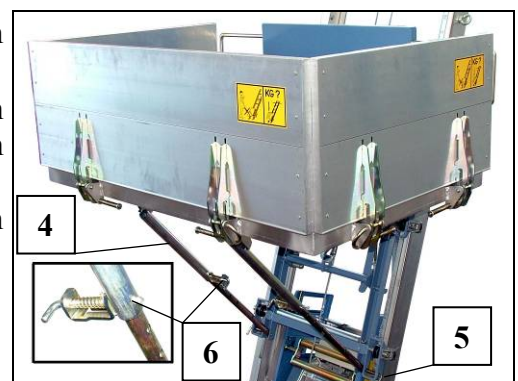
Fig. 51 Transportplateau
