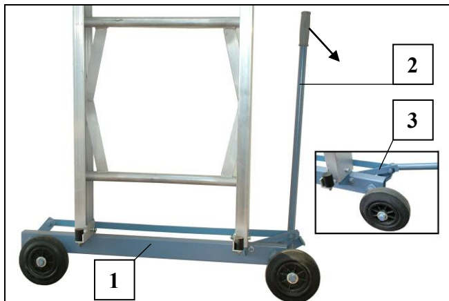
Fig. 14 Onderstel
