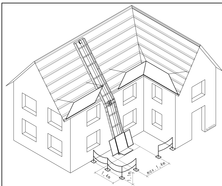
Fig. 3 Afzetten van de gevaarzone
