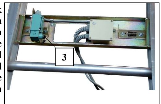
Fig. 70 Flexibele schakelaar
