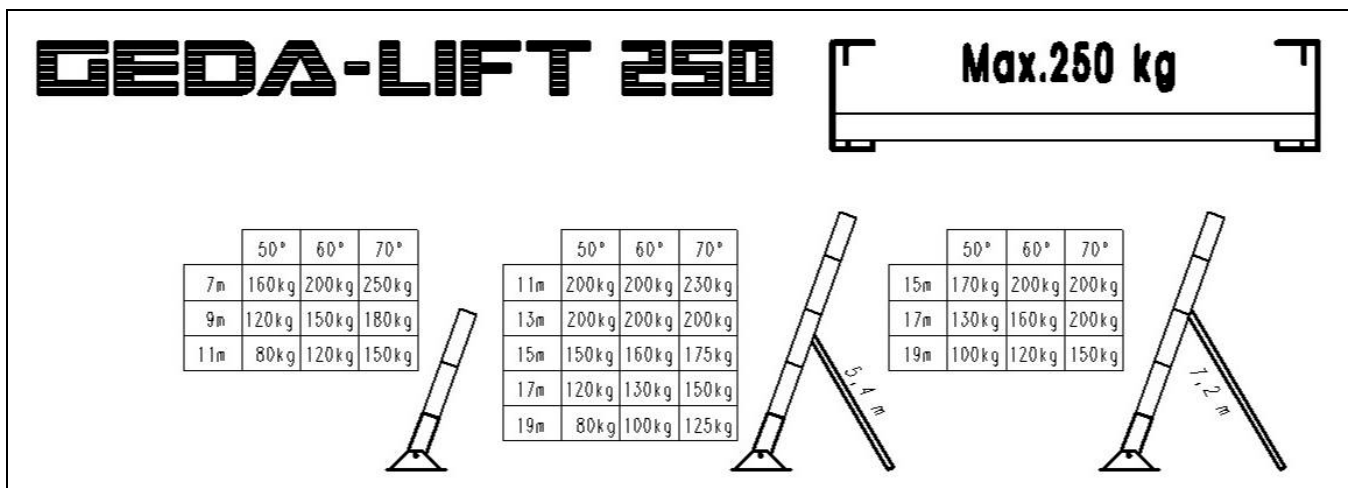
Fig. 25 Belastingtabel voor ladderdelen 200/250 kg
