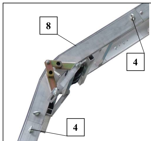
Fig. 21 Knikstuk monteren leggen en omhoogtrekken.
