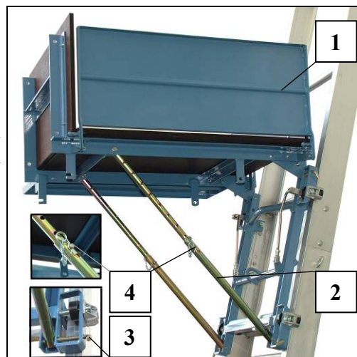
Fig. 47 Vario-platform
