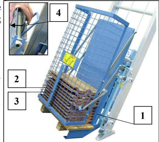
Fig. 56 Pannenplateau
